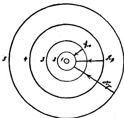
2. ábra. Hidrogénatomban keringő elektron 5 legbelső pályája 20 milliószoros nagyítással.
