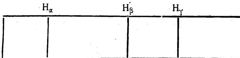
3. ábra. Az izzó hidrogén színeke normális nyomás mellett.
